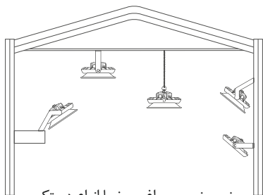
نحوه نصب چراغ مریخ با انواع دستک
